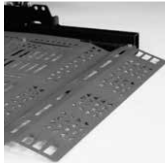
Plataforma autonivelante con revestimiento de tracción.
